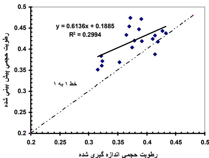
شکل ۲. مقایسه مقادیر اندازه‌گیری شده رطوبت حجمی در برابر مقادیر پیش‌بینی شده با مدل LEACHC در تیمار D1L1
