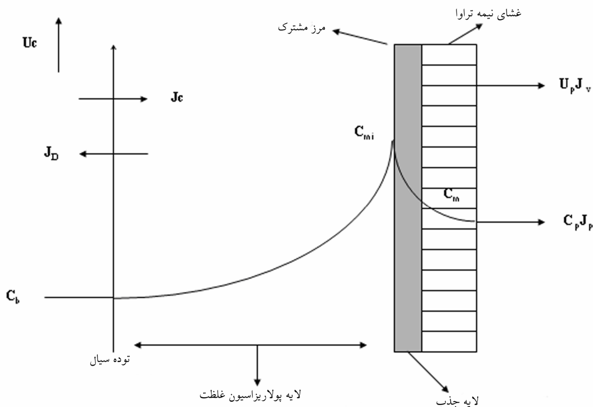
شکل ۱. شماتیک مقاومت‌های سر راه جریان در فرایند فرآپالایش جریان عرضی
