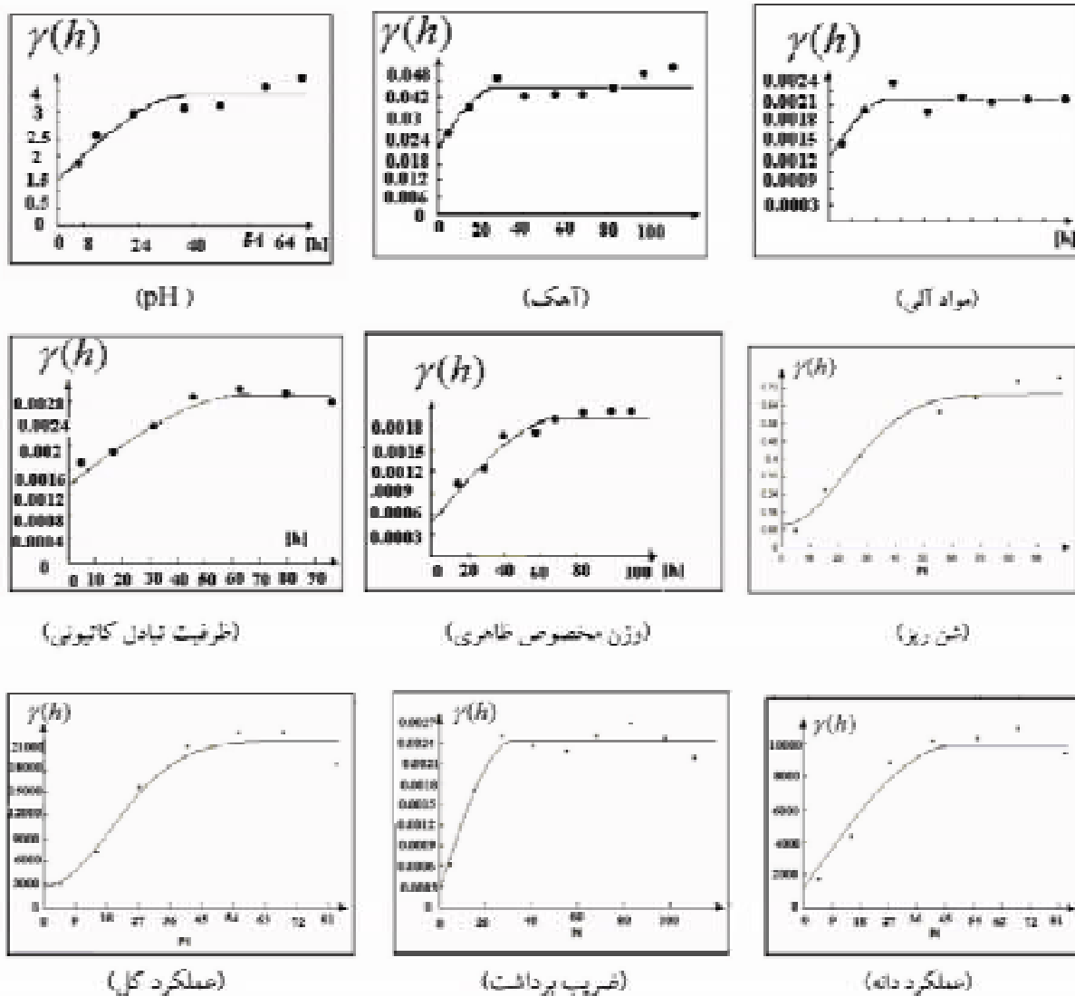
شکل ۲. تغییرنمای همه جهته برخی متغیرهای خاک و محصول
