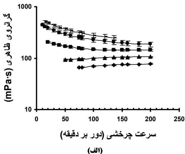
شکل ۲. نمایش رفتار جریان محلول‌های پودر ثعلب در غلظت‌های مختلف (۷، ۶، ۵، ۴، ۳، ۲ گرم در لیتر) در دمای ۲۵ درجه سانتی‌گراد و پ هاش ۷ الف) سرعت چرخشی در مقابل گرانیوی ظاهری ب) سرعت برشی در مقابل گرانیوی ظاهری.
