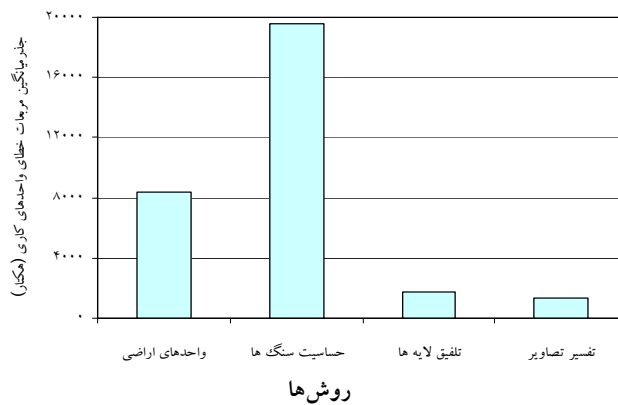
شکل ۲. جذر میانگین مربعات خطای واحدهای کاری روش‌های تهیه نقشه شکل‌های فرسایش
