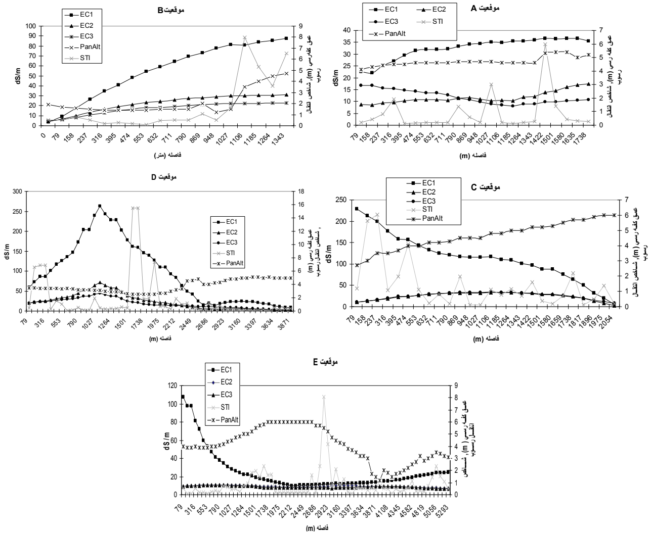
شکل ۸. نمودارهای ترانسکت‌ها در موقعیت‌های A، B، C، D و E و رابطه آنها با شوری ۵۰-۱۰۰ سانتی‌متر (EC1)، ۱۵۰-۱۰۰ سانتی‌متری خاک (EC2) (دسی‌زیمنس بر متر)، شاخص انتقال رسوب (STI) و عمق کفه رسی (PanAlt).
