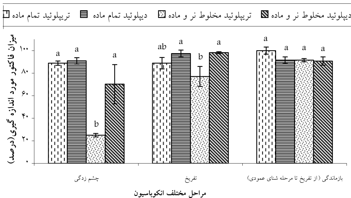
نمودار ۱. مقایسه نتایج حاصل از مرحله انکوباسیون تولید جمعیت تمام ماده تریپلوئید قزل‌آلای رنگین کمان
