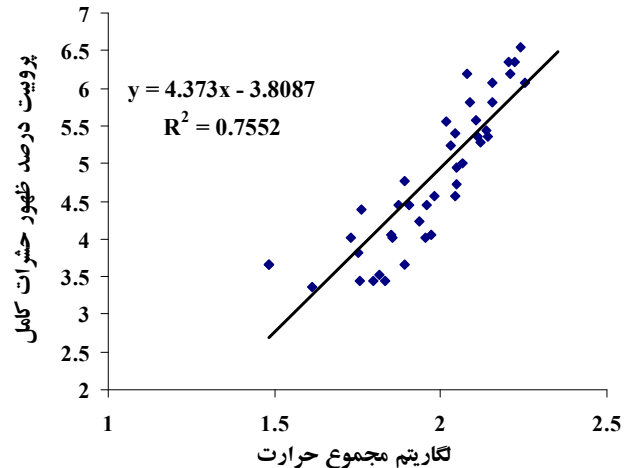
شکل ۱۰- رابطه خطی بین پرویت درصد ظهور حشرات کامل پروانه چوبخوار پسته و لگاریتم مجموع حرارت مؤثر از ۵۰ درصد تشکیل پيله شفيرگی تا ظهور حشرات کامل براساس آستانه حداقل حرارتی ۱۲ درجه سانتی‌گراد در شرایط صحرائی
