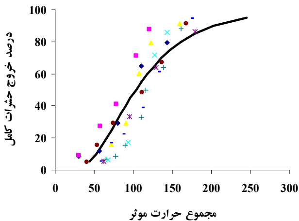
شکل ۱۱. مجموع حرارت مؤثر لازم برای درصد‌های ظهور حشرات کامل پروانه چوبخوار پسته از ۵۰ درصد تشکیل پيله شفيرگی براساس آستانه حداقل حرارتی ۱۲ درجه سانتی‌گراد در شرایط صحرائی
