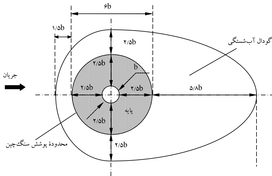
شکل ۱۲. ابعاد نهایی گودال آب‌شستگی دور تک پایه دارای سنگ چین با قطر ۲/۸۶ میلی‌متر در حالت U/U_c = ۰/۹۵
