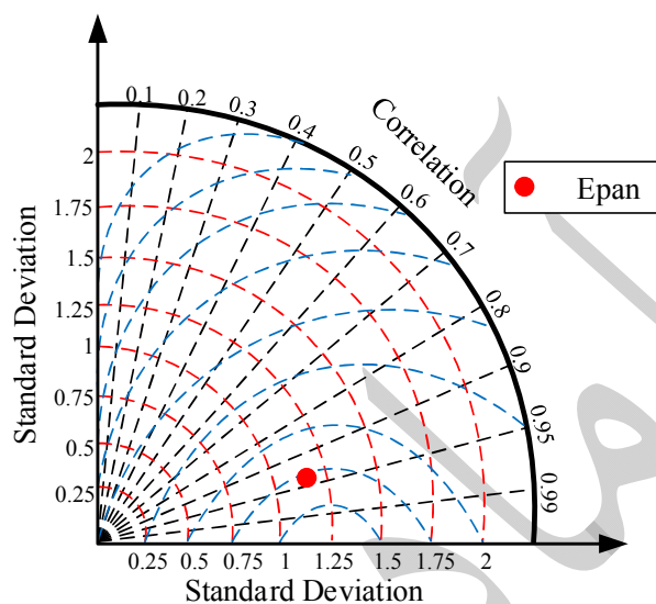
شکل ۱۱. دیاگرام تیلور
