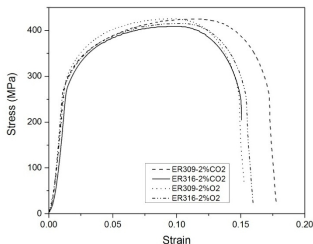
شکل ۱۱- منحنی‌های تنش - کرنش نمونه‌های جوشکاری شده.
