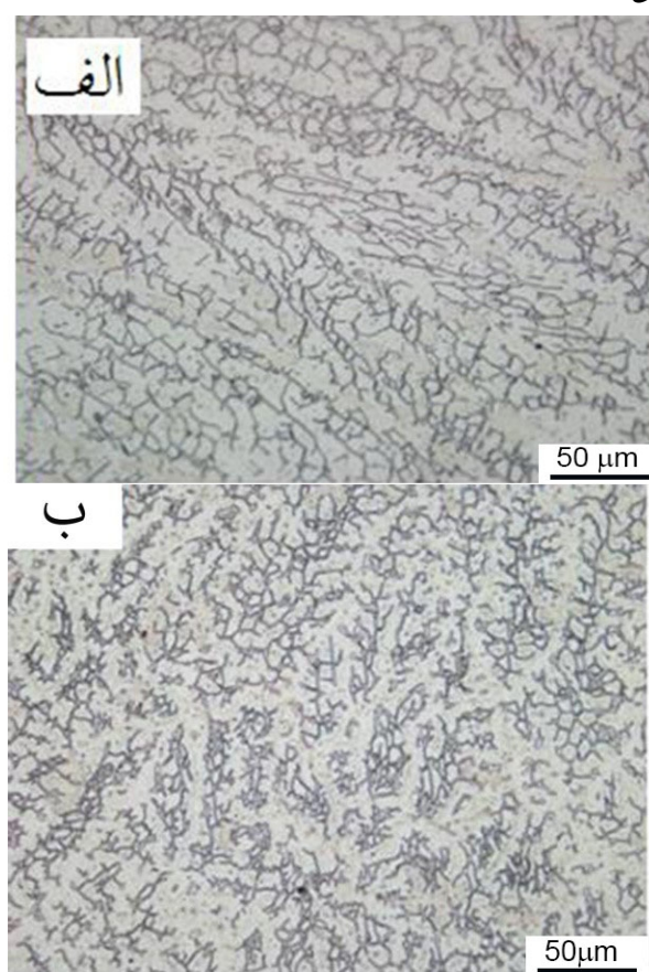
شکل ۸- تصویر میکروسکوپی نوری منطقه جوش: (الف) نمونه ۱ و (ب) نمونه ۳.
