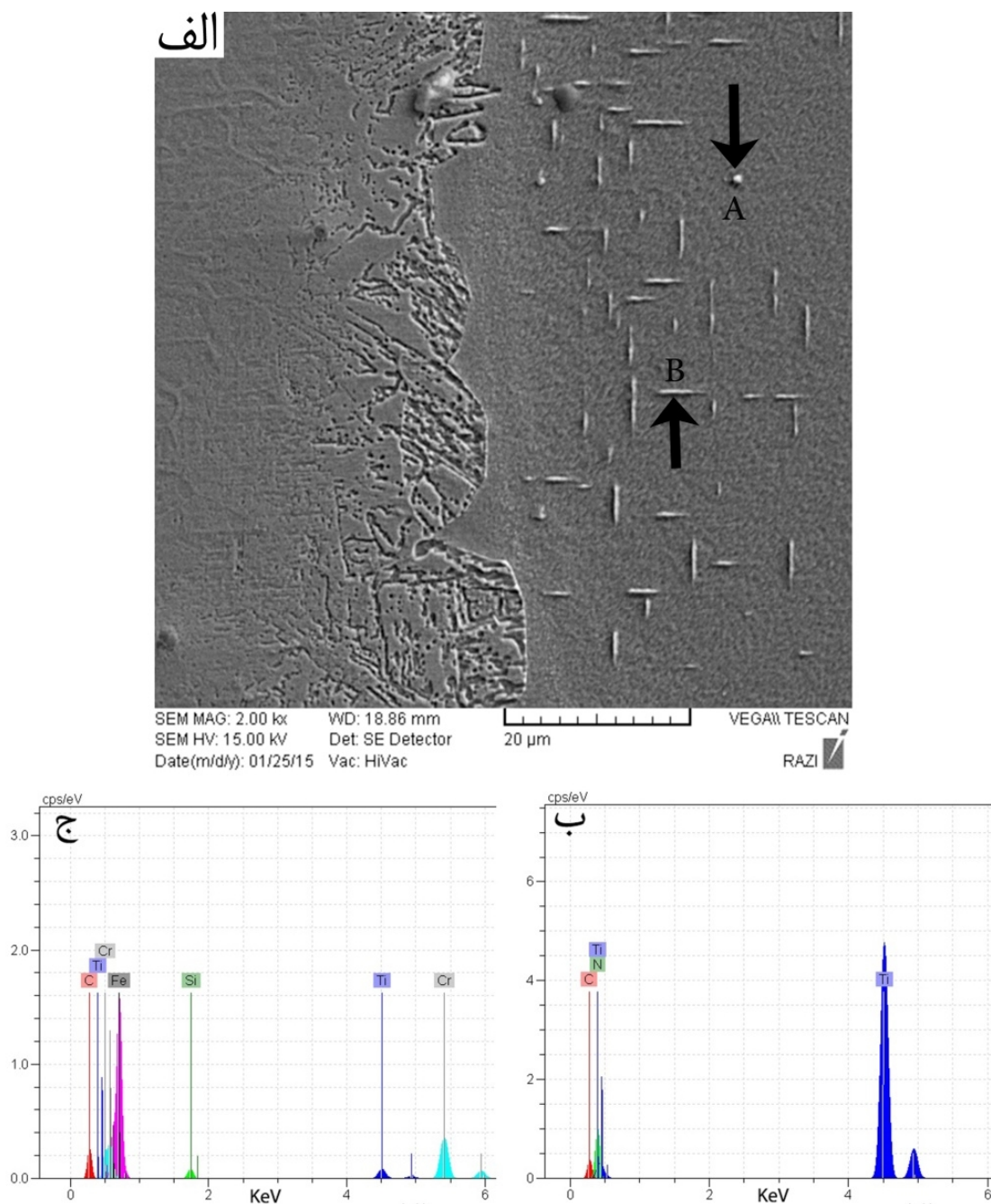
شکل ۱۰- (الف) تصویر میکروسکوپی الکترونی روبشی منطقه تحت تاثیر حرارت فلز پایه ۴۰۹ نمونه ۴،
