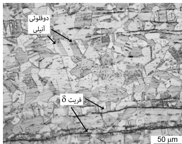
شکل 1- تصویر میکروسکوپی نوری از ریزساختار فلز پایه فولاد آستیتی 304 L (فريت δ و دوقلوئی های آنیلی با پیکان مشخص شده اند).
