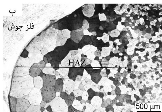
شکل ۹- تصویر میکروسکوپی نوری از ریز ساختار منطقه تحت تاثیر حرارت فلز پایه نمونه ۱: (الف) فولاد فریتی ۴۰۹ و (ب) فولاد آستنیتی ۳۰۴L.
