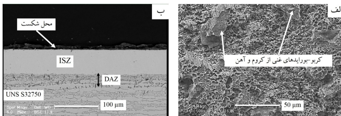
شکل 7- تصویر میکروسکوپ الکترونی روبشی از (الف) سطح شکست نمونه های متصل شده در دمای 1050 درجه سانتی گراد به مدت 45 دقیقه و (ب) سطح مقطع نمونه شکسته شده.
