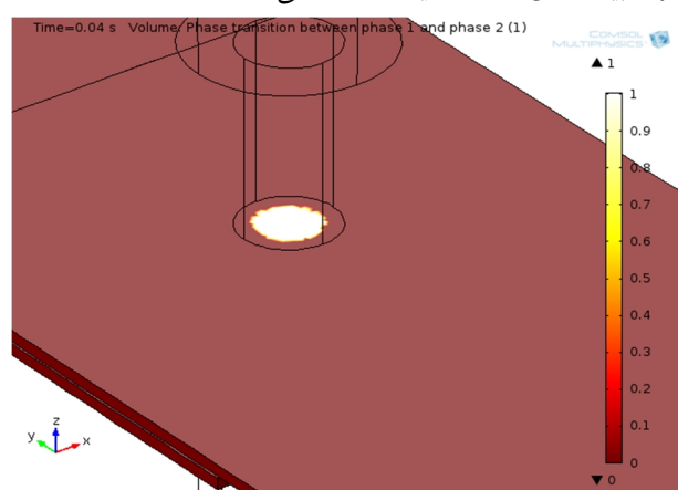
شکل 4- شبیه سازی مدل جدید (40Ms، 1000A و 100N)
