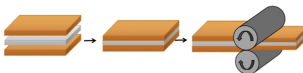
شکل 1- شمای کلی فرایند نورد سرد پیوندی برای سه لایه، شامل دو لایه برنج در اطراف و یک لایه فولاد در وسط.
