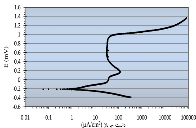
شکل 2- منحنی آزمون خوردگی پلاریزاسیون سیکلی فلز پایه در محلول 0.5M H 2 SO 4
