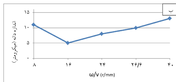
شکل 9- رابطه متوسط اندازه دانه با نسبت سرعت چرخشی به سرعت پیشروی در نمونه های جوشکاری شده: الف) بدون استفاده از لایه میانی AA7075 ب) با استفاده از لایه میانی AA7075.
