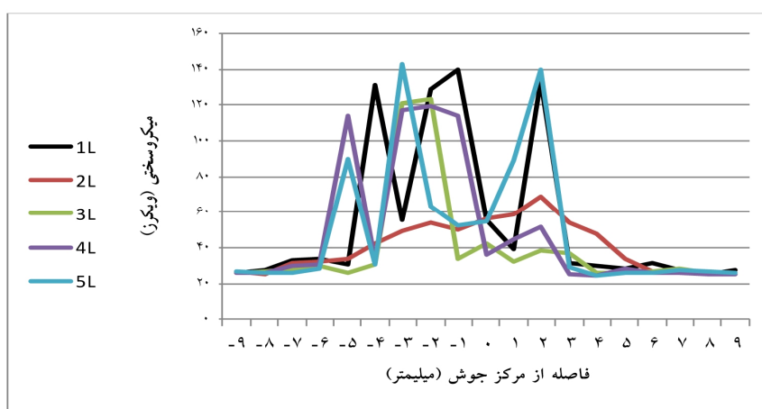
شکل 13- نمودار ریزسختی منطقه جوش در فاصله 2/5 میلی متر پایین تر از سطح جوش در نمونه های با لایه واسط، الف) نمونه های 1L، 2L، 3L، 4L، 5L.
