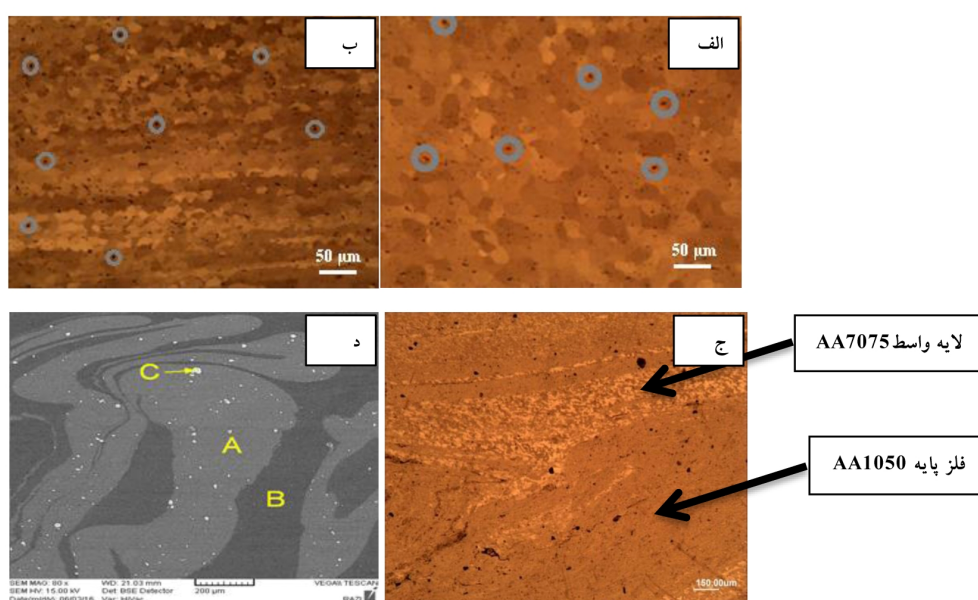
شکل 4- تصاویر الف) ناحیه اغتشاش نمونه 1، ب) ناحیه اغتشاش نمونه L1، ج) نواحی لایه ای نمونه L1 و د) SEM از نمونه L1.
