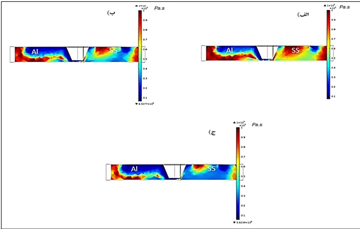
شکل ۱۴- کانتورهای توزیع گرانی دینامیکی در عرض مقطع جوش در سرعت های چرخشی متفاوت. سرعت 350 RPM (الف)، سرعت 500 RPM (ب) و سرعت 700 RPM (ج)
