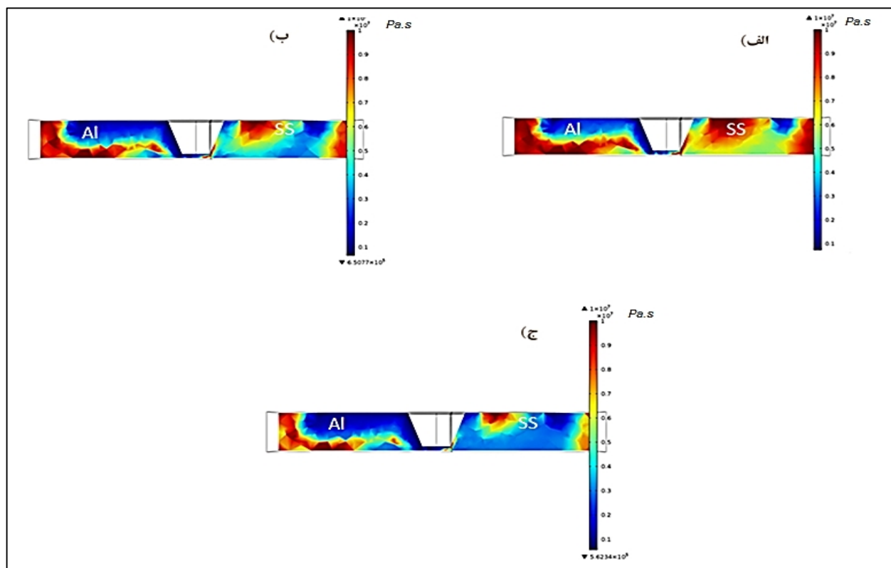
شکل ۱۴- کانتورهای توزیع گرانیروی دینامیکی در عرض مقطع جوش در سرعت های چرخشی متفاوت. سرعت 350 RPM (الف)، سرعت 500 RPM (ب) و سرعت 700 RPM (ج)
