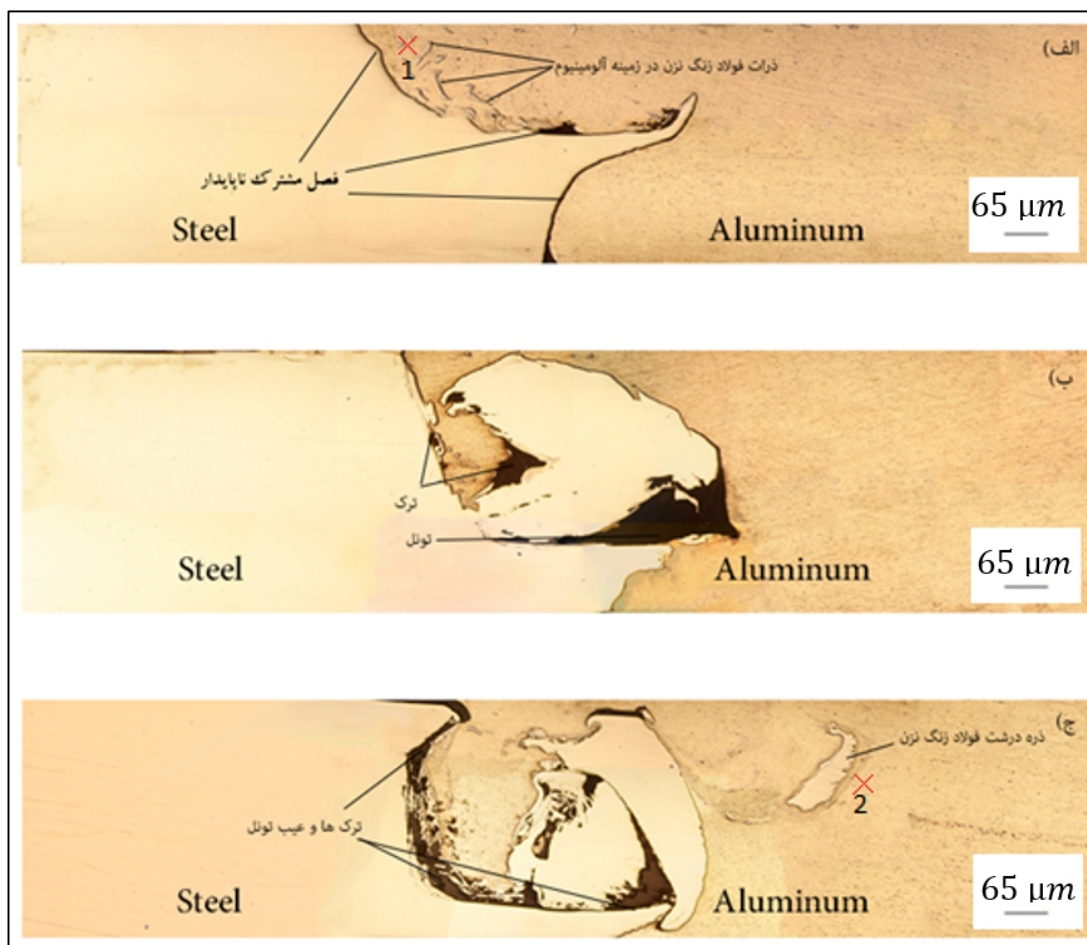
شکل ۵- تصویر میکروسکوپی نوری اتصال فولاد زنگ نزن به آلومینیوم در سرعت الف) RPM350.
