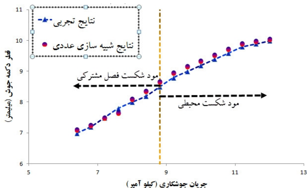
شکل ۱۲ - نتایج تجربی و شبیه سازی عددی تأثیر جریان جوشکاری بر اندازه دکه جوش و مود شکست
