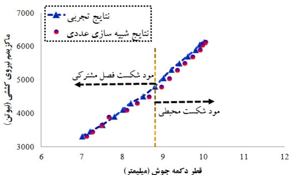
شکل ۱۳ - نتایج تجربی و شبیه سازی عددی تأثیر قطر دکه جوش بر ماکزیمم نیروی کششی جوشهای نقطه ای مقاومتی
