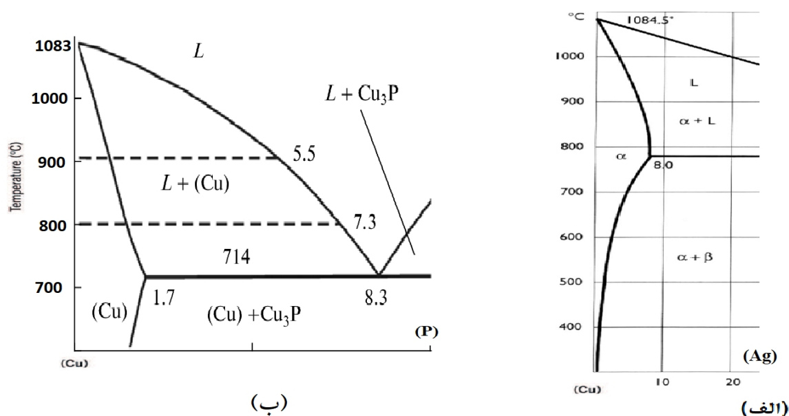
شکل 11- دیاگرام های فاز می - نقره و مس - فسفر: الف) دیاگرام فاز می - نقره و مس - فسفر و ب) دیاگرام فاز می - مس - فسفر
