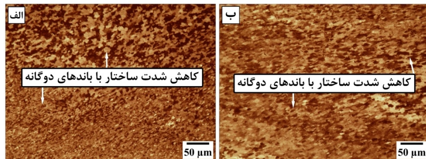
شکل 13- ساختار با باندهای دوگانه در ناحیه تلاطم یافته در سه پاس فرایند FSW و در الف- \omega/v=25 r/mm و ب- \omega/v=70 r/mm.
