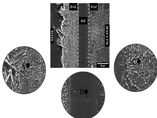
شکل 4- تصویر میکروسکوپ الکترونی روبشی (SEM) اتصال انجام شده در دمای 1150 درجه سانتی‌گراد و زمان 5 دقیقه
