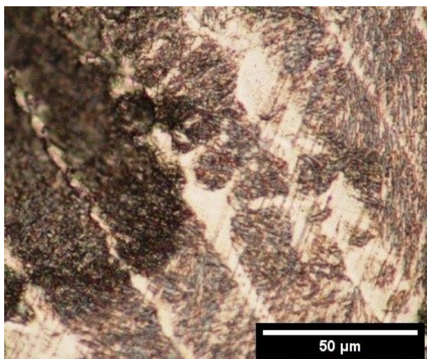
شکل 4- تصویر میکروسکوپ نوری فلز جوش حاصل از پرکننده ER309L بر روی فلز پایه قبل از نیتروژن‌دهی.
