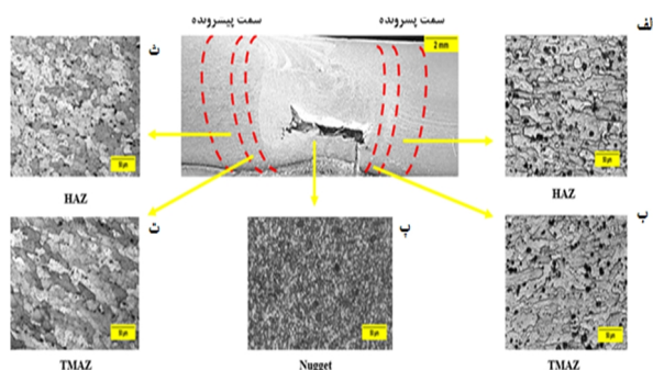
شکل 5- مقطع عرضی نمونه شماره 4 (سرعت چرخشی 600 rpm و سرعت پیشروی 90 mm/min) و تصویر میکروسکوپی منطقه الف- ناحیه متأثر از حرارت در سمت پسرونده، ب- ناحیه متأثر از عملیات ترمومکانیکی در سمت پسرونده، پ- ناحیه اغتشاشی دکمه جوش، ت- ناحیه متأثر از عملیات ترمومکانیکی در سمت پیشرونده، ث- ناحیه متأثر از حرارت در سمت پیشرونده.
