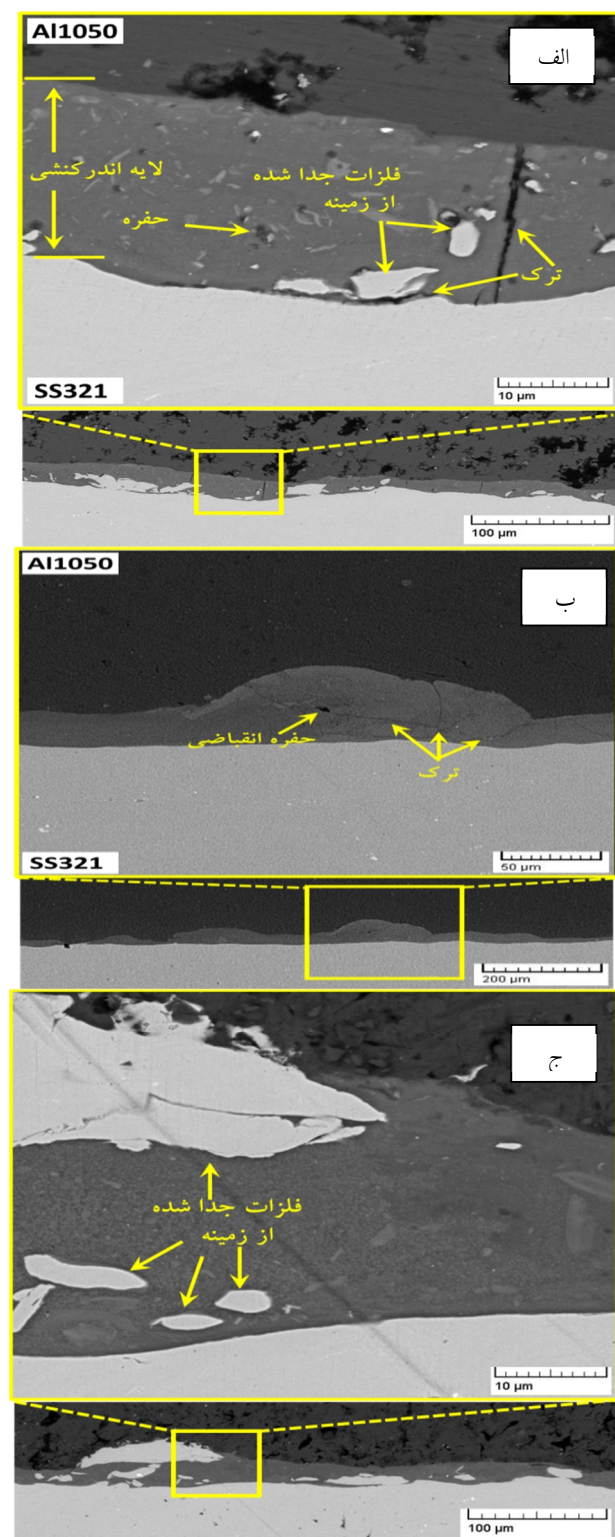
شکل 3- تصویر میکروسکوپ الکترونی لایه واکنشی در فصل مشترک Al1050-SS312 اتصال 3 لایه الف و ب- نمونه بعد از جوشکاری، ج- نمونه عملیات حرارتی شده در دمای 250 درجه سانتی گراد.
