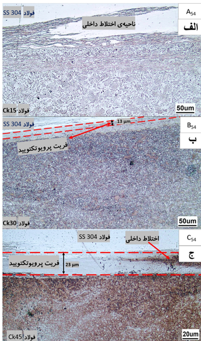
شکل 6- تصاویر میکروسکوپ نوری از ریزساختار ناحیه جوش سه نمونه الف - A_{54} ، ب - B_{54} و ج - C_{54} در سمت ساده کربنی.
