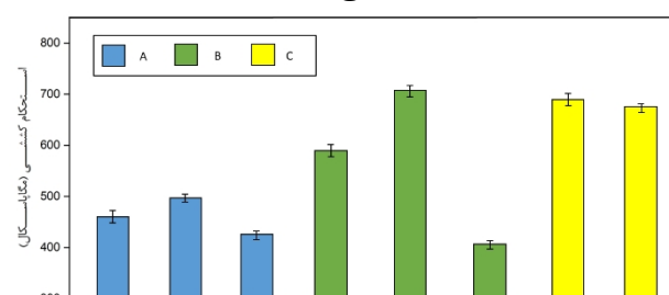
شکل 5- نتایج آزمایش کشش انجام گرفته بر روی تمامی نمونه‌های سری A، سری B و سری C.
