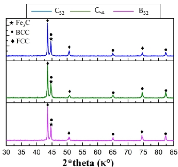
شکل 12- نتایج آزمایش پراش پرتو ایکس نمونه C 52 , C 54 و B 52 .
