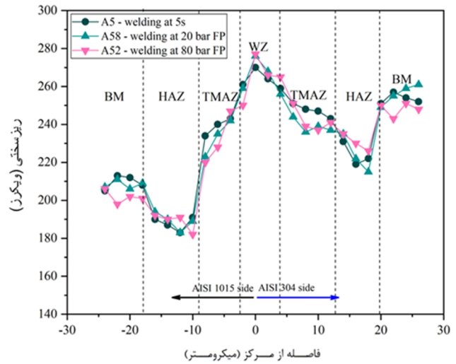
شکل 13- نتایج آزمایش ریزسختی بر روی نمونه‌های سری A.
