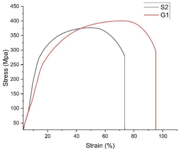
شکل 21- نمودار تنش- کرنش نمونه‌های آزمون کشش: G1 - GMAW، S2 - SMAW.
