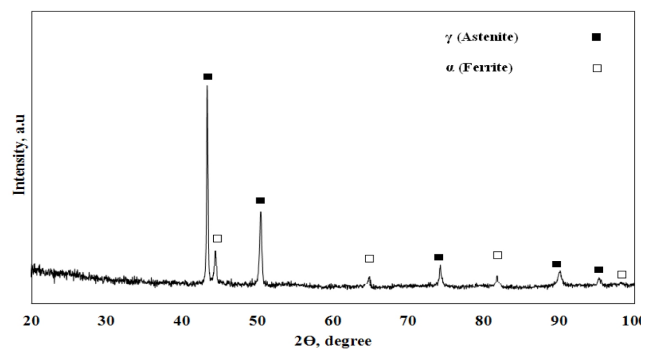
شکل 10- الگوی پراش پرتو ایکس از منطقی مجاور جوش نمونه‌های حاصل از جوشکاری تحت عملیات پیش‌گرمایش 100 درجه سانتی‌گراد.
