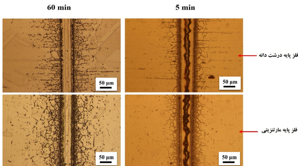
شکل ۹- ریزساختار منطقه اتصال فاز مایع گذرا در فولاد زنگ نزن L ۳۰۴ با دو ساختار آستنیتی درشت دانه و مارتنزیتی
