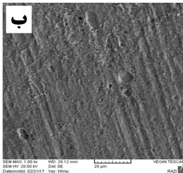
شکل 6- تصاویر میکروسکوپ الکترونی روبشی از سازوکار خوردگی فلز جوش ایجاد شده با حرارت ورودی: الف) 12/6 kJ/mm ، ب) 37/8 kJ/mm
