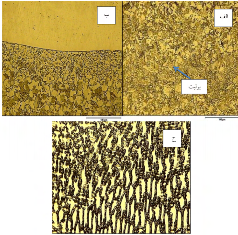
شکل 3- تصویر OM نمونه روکشکاری و عملیات حرارتی شده. الف) BM عملیات حرارتی شده در 750 درجه سانتیگراد، ب) نمونه عملیات حرارتی شده در 850 درجه سانتی گراد و ج) کاربدهای منطقه CL عملیات حرارتی شده 850 درجه سانتی گراد
