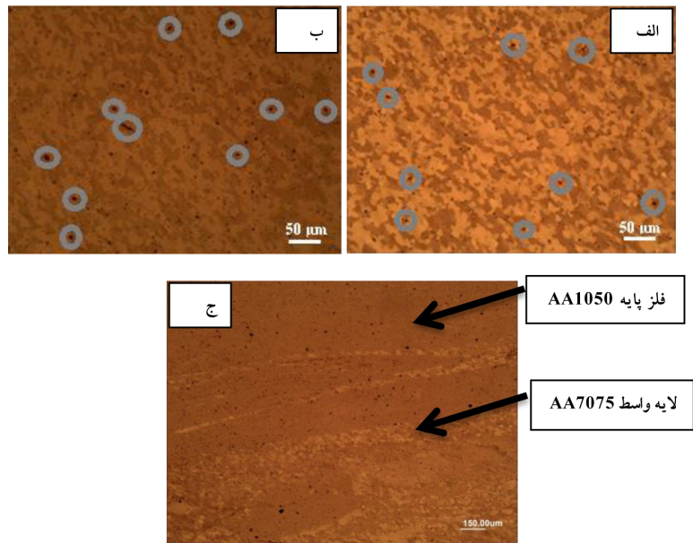
شکل 5- تصویر الف) ناحیه اغتشاش نمونه 2، ب) ناحیه اغتشاش نمونه 2L، ج) نواحی لایه ای نمونه 2L.
