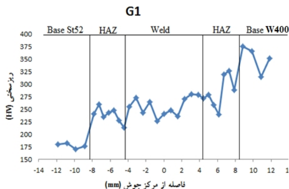
شکل 10- تغییرات ریزسختی در جوش، منطقه متأثر از حرارت و فلز پایه نمونه G1.
