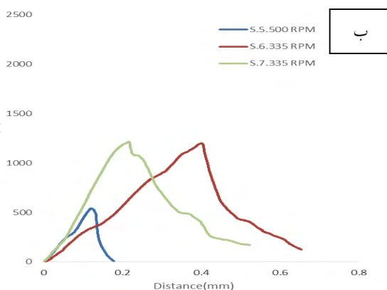
شکل ۲-الف) استحکام کششی برای فرایند لحیم کاری بدون روانساز و ابزار چرخشی، (ب) با روانساز.
