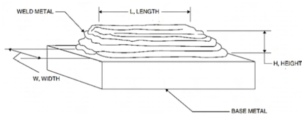
شکل ۲- شماتیک نمونه کوآتومتری مناسب جهت تعیین ترکیب شیمیایی
