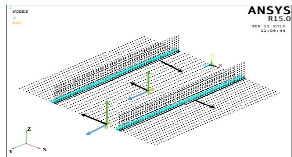
شکل ۶- شرایط مرزی اعمال شده بر روی پانل
