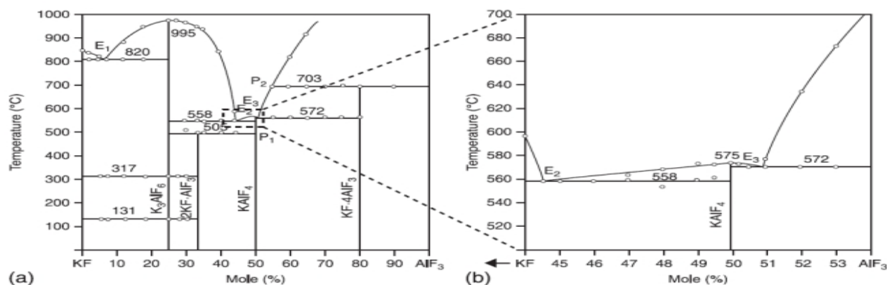
شکل 6- دیاگرام فازی KF-AlF_3 [19].
