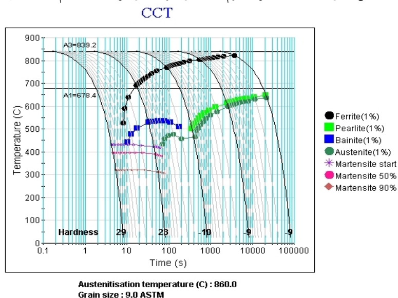
شکل 5- نمودار CCT فولاد DP590 به کمک نرم افزار شبیه سازی JMat
