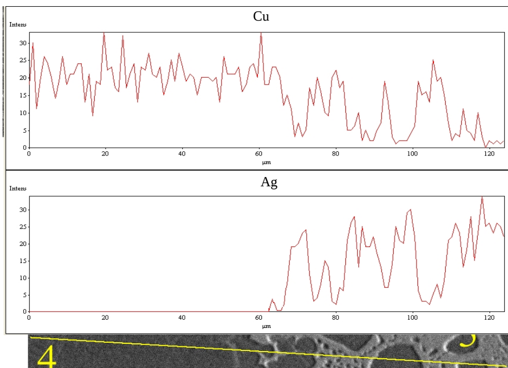
شکل 13- نسبت حضور مس و نقره در مقطع جوش با پرکننده Cu-Ag-P
