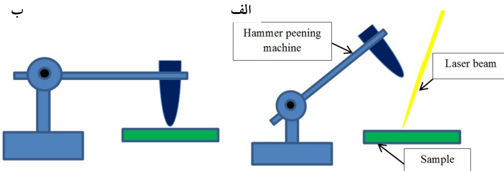
شکل 7- توالی لیزر و کوبش. الف) پرتو لیزر به سطح قطعه کار تابانده شده است و ب) کوبش در ناحیه اعمال پرتو لیزر انجام شده است.
