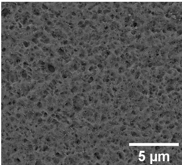
شکل 8- تصویر ریزساختار آلیاژ در مرکز اتصال.
