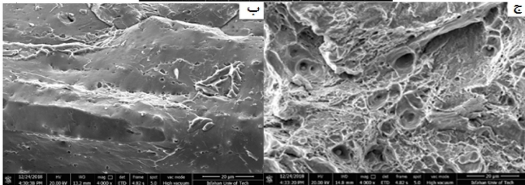
شکل 9- تصاویر میکروسکوپی الکترونی روبشی از سطح شکست نمونه‌های جوشکاری شده پس از آزمون کشش
