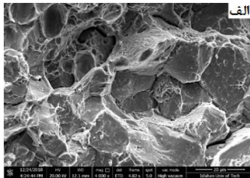
شکل 8- تصویر ناحیه شکست نمونه‌های جوشکاری لیزری شده پس از آزمون کشش.
