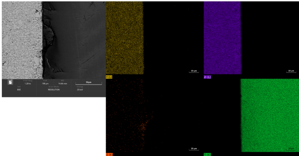
شکل 5- نتایج آنالیز Map از ناحیه ترک خورده در فصل مشترک Ti/3YSZ در دمای 960^{\circ}\text{C} و زمان 20 دقیقه
