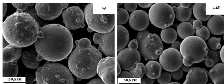
شکل 1- الف- تصویر میکروسکوپی الکترونی روبشی پودر استالایت 6061 ب- تصویر میکروسکوپی الکترونی روبشی پودر فولاد زنگ‌نزن 4PH-17.
