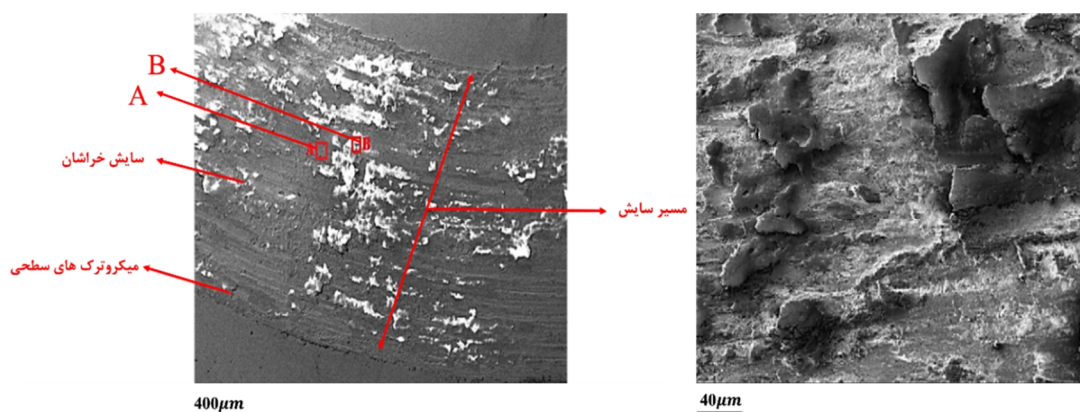
شکل 8- تصویر میکروسکوپی الکترونی رویشی از مسیر سایب روکش در دمای محیط.
