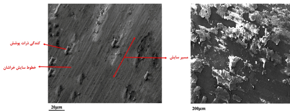
شکل 7- تصویر میکروسکوپی الکترونی رویشی از مسیر سایب زیرلایه در دمای محیط.
