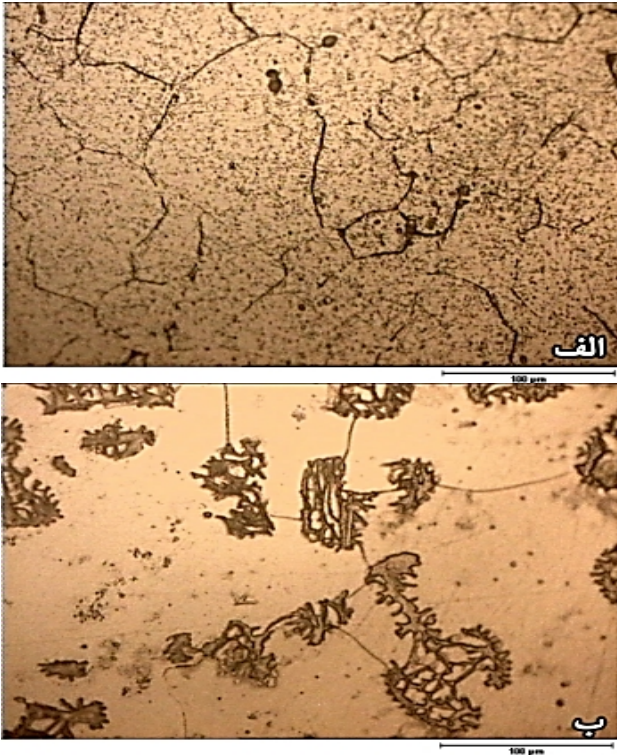
شکل 1- ریزساختار فلزات پایه (الف) سوپراآلیاژ (در دمای °C 1170 به مدت 30 دقیقه آبیل و در آب کوئچ شده) (ب) ترکیب بین فلزی Ni 3 Al.
