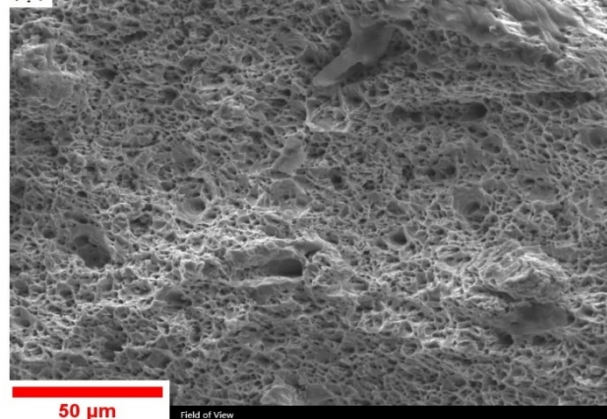
شکل 18- تصویر شکست نگاری از سطح مقطع شکست فولاد AISI 430 در دو بزرگنمایی متفاوت.
