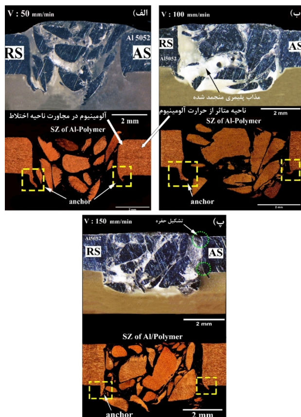
شکل 3- تغییرات اندازه لنگر در نمونه‌های الف-50T، ب-100T و پ-150T.
