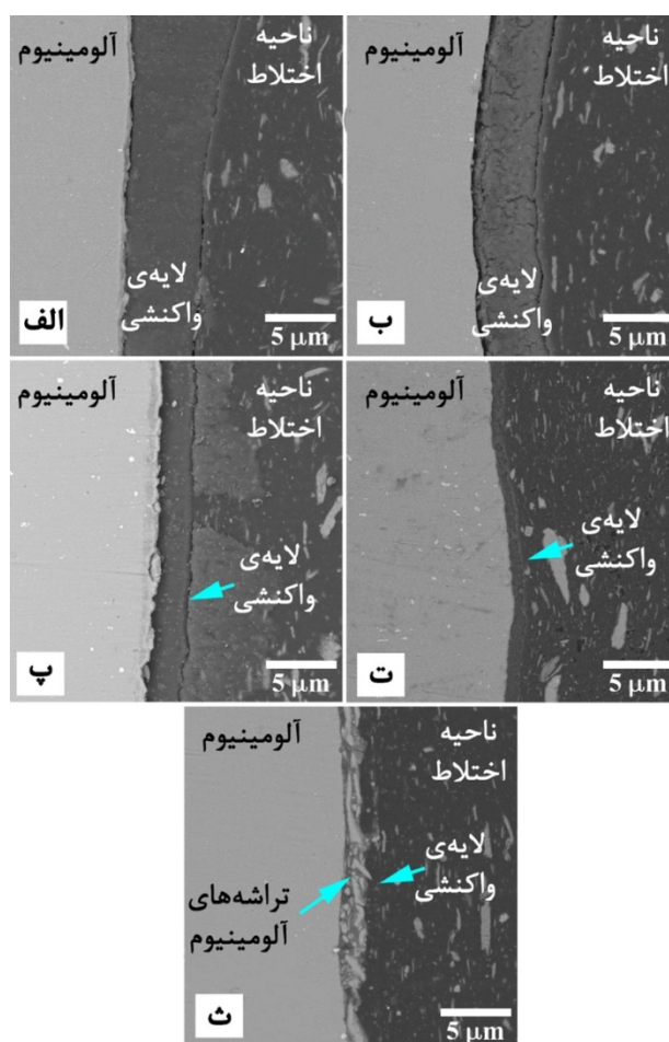
شکل 6- تغییرات لایه واکنشی در نمونه‌های الف - 300R - ب - 500R
