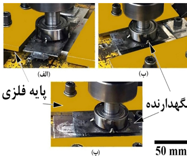
شکل 2- نحوه استفاده از پایه فلزی و نگه‌دارنده جهت جوشکاری نمونه‌ها از زوایای مختلف.
