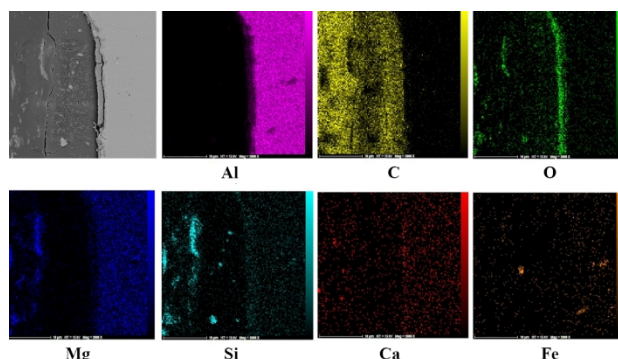
شکل 7- نقشه توزیع عنصری در لایه واکنشی نمونه‌ها.
