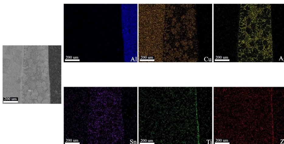
شکل 13- آنالیز نقشه عنصری از تصویر ریزساختار اتصال \text{Al}_2\text{O}_3/\text{Cu} با فلز پرکننده Ag-Cu-Ti-Sn-3.5Zr.
